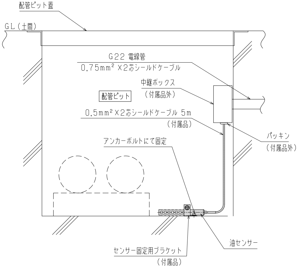
配管ピット内設置図
